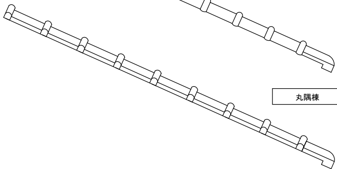
三角隅棟
