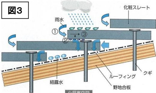
化粧スレートの小口面①と裏面②から化粧スレート内③へ浸透
